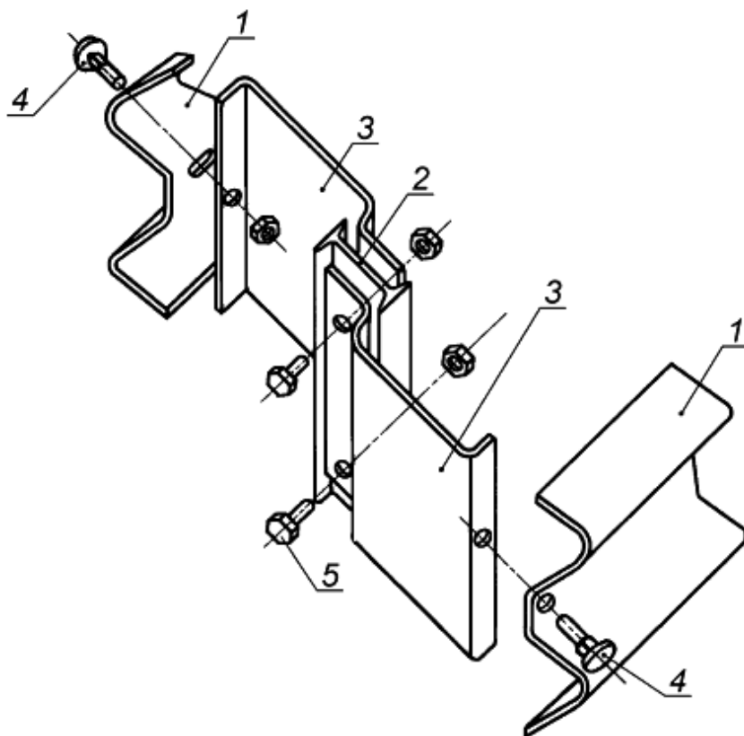
Рисунок А.3 - Одностороннее ограждение мостовой и дорожной групп с консолью-амортизатором. Соединение балки со стойкой
