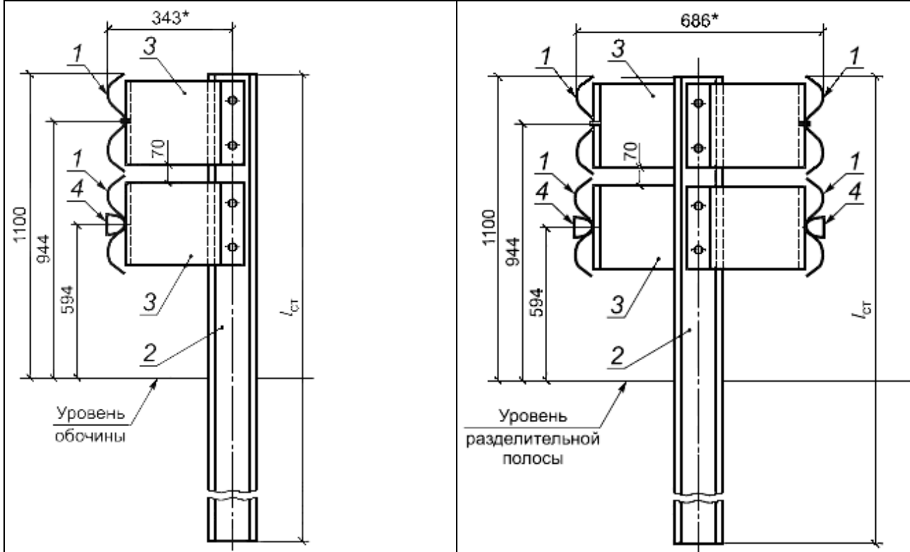
в) Одностороннее двухъярусное ограждение г) Двухстороннее двухъярусное ограждение
