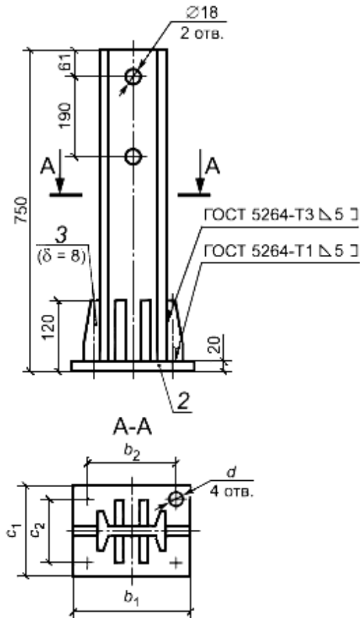
Рисунок 9 - Консоль-распорка КР
