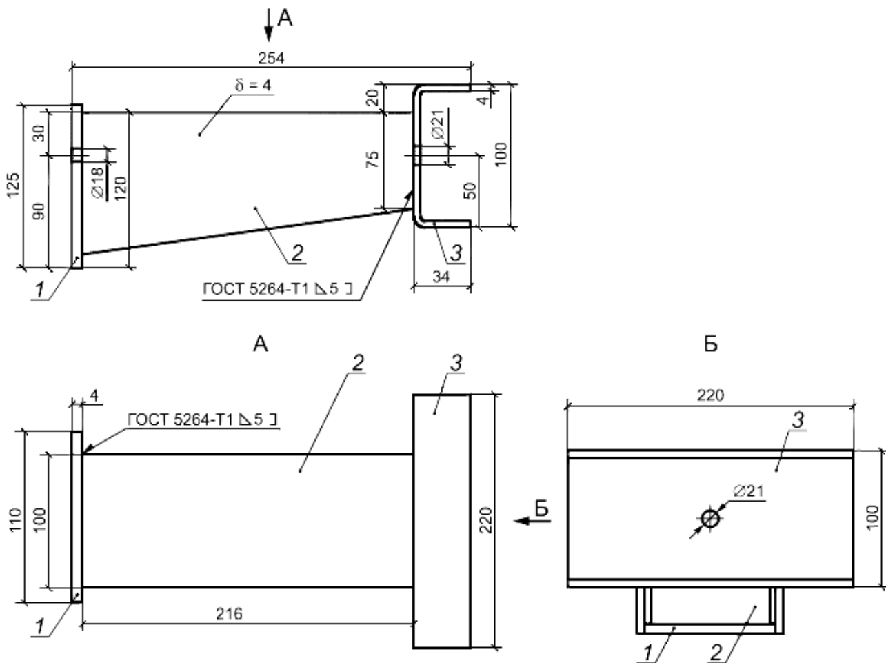
Рисунок 7 - Стойки дорожные СД
