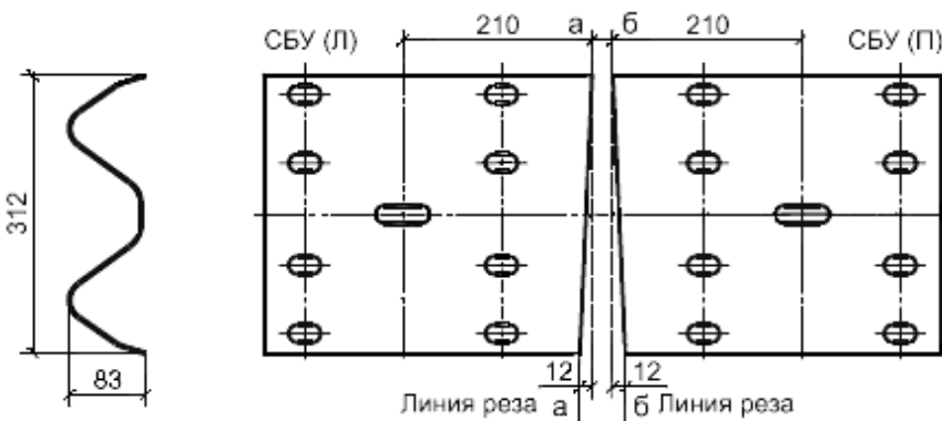
Рисунок 4 - Секция балки ограждений СБ
