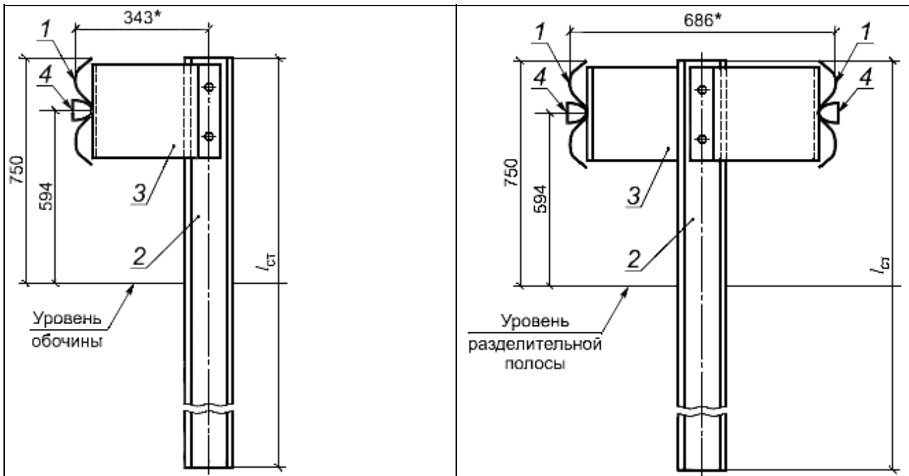
а) Одностороннее одноярусное ограждение б) Двухстороннее одноярусное ограждение
