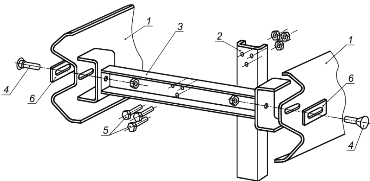
Рисунок А.1 - Одностороннее ограждение дорожной группы с жесткой консолью. Соединение балки со стойкой
